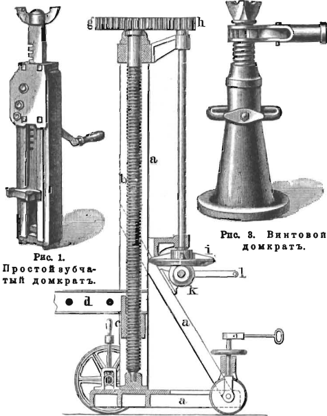
Рис. 2. Домкратъ для поднятія паровозовъ.
