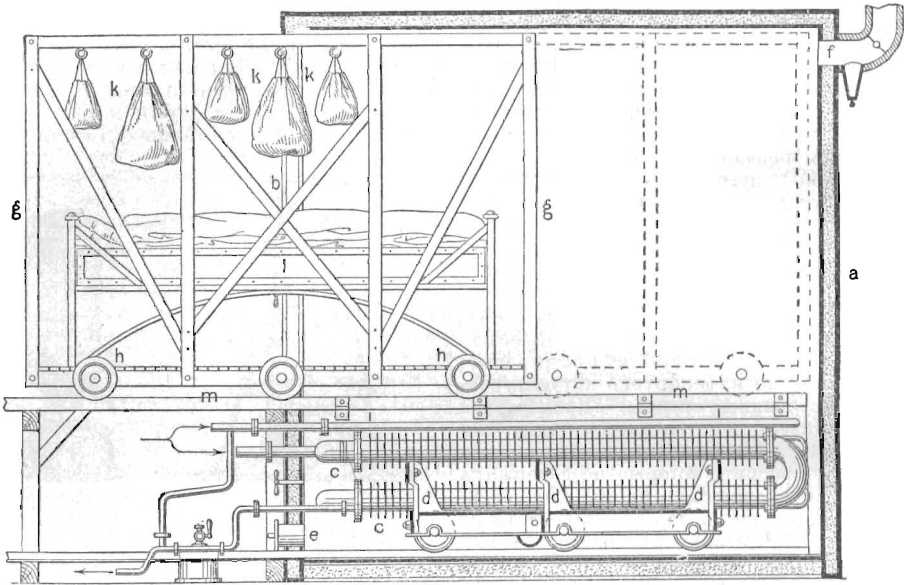
Фиг. 3. Желѣзный дезинфекціонный аппаратъ. а двойная стѣна; б дверь, въ которую въдвигается на колесахъ h по длинѣ шинъ m телѣжка g съ предназначенными для дезинфекціи вѣшами; с мѣдныя спирали для точки.
