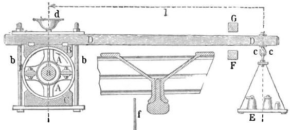
Фиг. 1. Тормазный динамометръ Прони.
