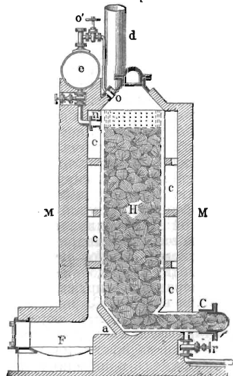
Рис. 2. Котелъ для вывариванія дерева въ натронномъ щелоѣ.
