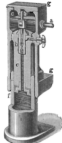
Рис. 4. Гидравлическій домкратъ.
