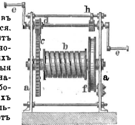
Рис. 5. Простой домкратъ.
