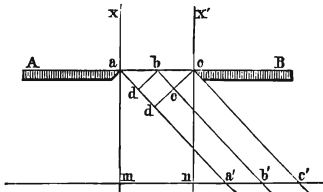
Фиг. 2. Объясненіе диффракціи.
