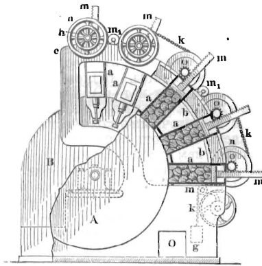
Рис. 1. Древоотерка Фельтера.
