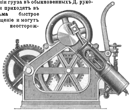
Рис. 6. Паровой домкратъ.
