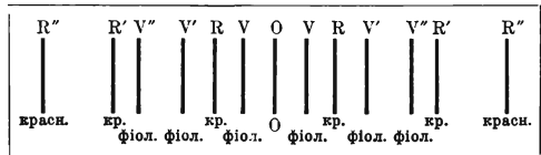
Фиг. 3. Образованіе спектровъ въ диффракціонныхъ сѣткахъ.
