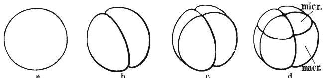
Фиг. 2. Неравномерное дробленіе яйца лягушки.
