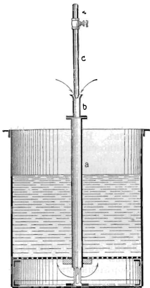
Фиг. 17. Гаргривовъ (Hargreaves) приборъ для окисленія.
