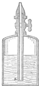
Героновъ шаръ.
