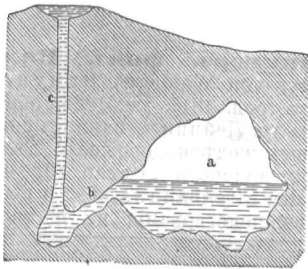
Фиг. 3. Схема гейзера по Мэкензи.
