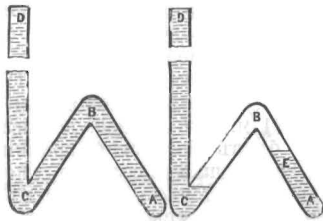
Фиг. 5. Къ теоріи гейзера по Лангу.
