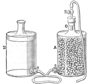
Фиг. 5. Газоотдѣлительный приборъ Девилла.
