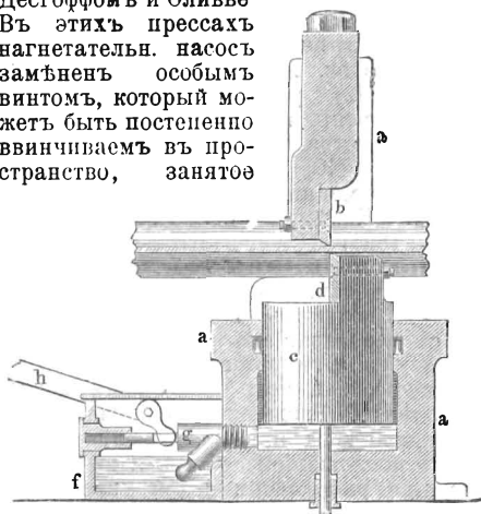
Рис. 2. Гидравлическія ножницы.
