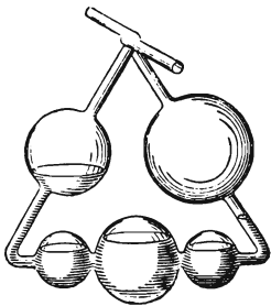
Фиг. 15. Кали-аппаратъ Либиха.
