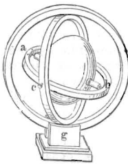
Фиг. 2. Приборъ Бененбергера.
