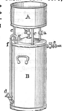
Фиг. 11. Газометръ лабораторный.
