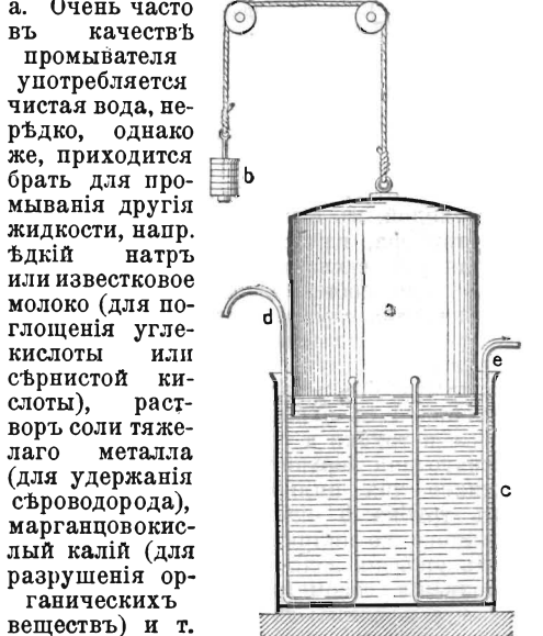
Фиг. 12. Газометръ или газгольдеръ.
