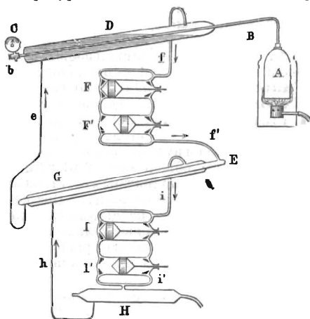
Приборъ Пикте для полученія жидкаго кислорода.
