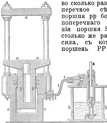
Рис. 1. Гидравлическій прессъ (разрѣзъ).
