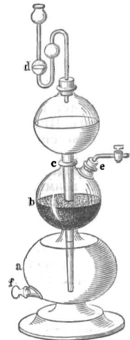
Фиг. 6. Газоотдѣлительный приборъ Киппа.
