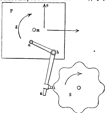
Фиг. 1. Гильошировальный приборъ.
