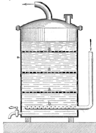
Фиг. 9. Промывательный сосудъ.
