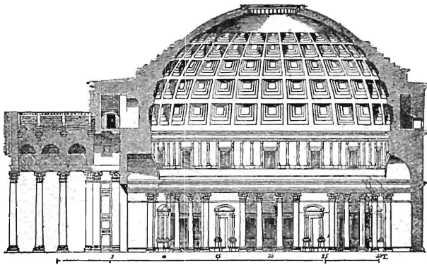
Рис. 8-й. Пантеонъ Римскій.
