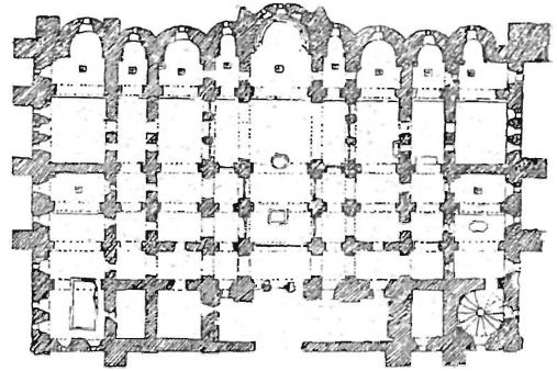
Рис. 25-й. Планъ Кіево-Софійскаго собора.
