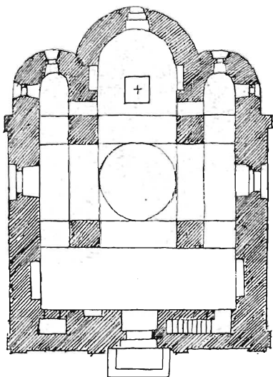
Рис. 30-й. Планъ неболъш. Новг. храма.
