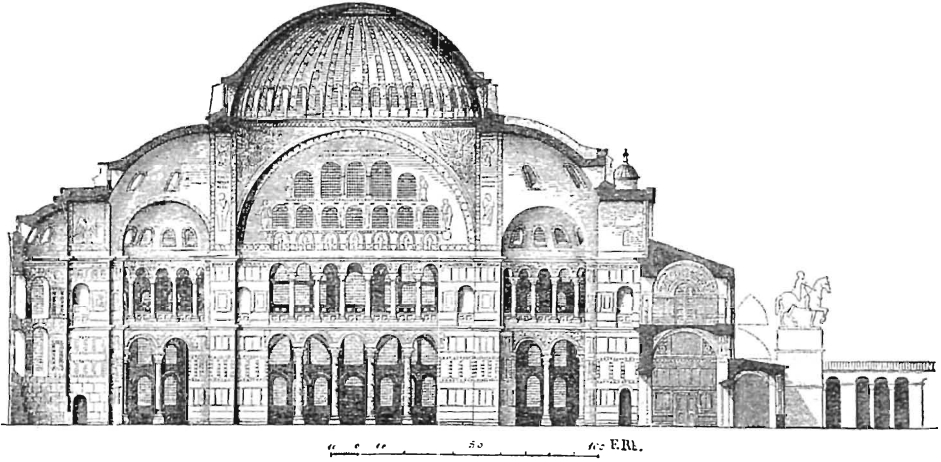
Рис. 10-й. Разрѣзъ храма св. Софіи въ Константинополѣ.
