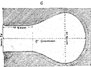
Рис. 34-й. Разрѣзъ такъ назыв. голосника.
