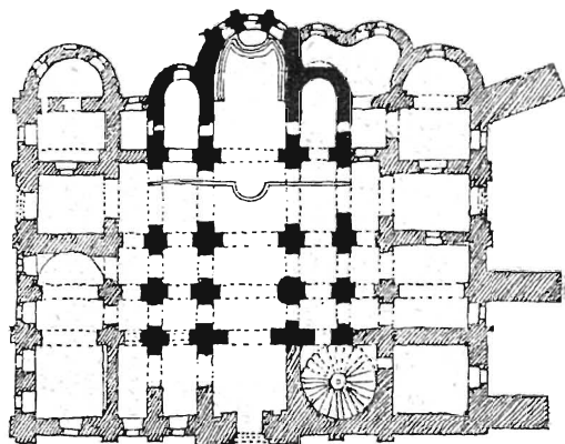
Рис. 29-й. Планъ Новгородскаго Софійскаго собора.
