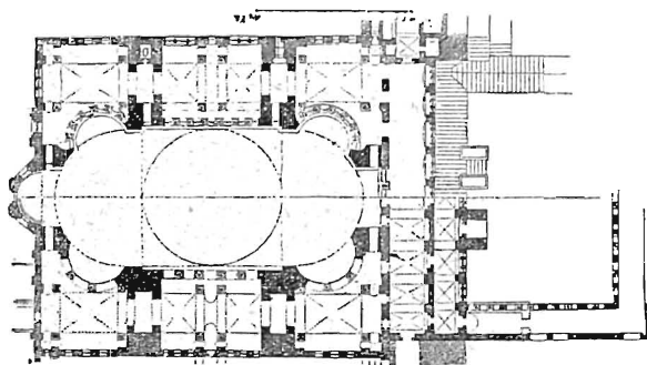
Рис. 16-й. Планъ храма св. Софїи въ Константинополѣ.
