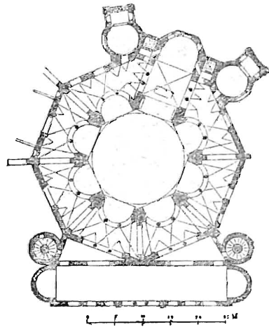
Рис. 14-й. Планъ храма св. Виталія въ Равеннѣ.
