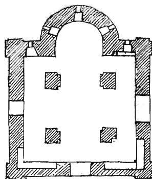
Рис. 31-й. Планъ маленькаго Новгородскаго храма.
