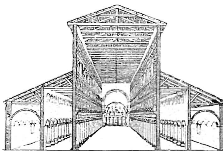
Рис. 4-й. Разрѣзъ древне-христіанской базилики.
