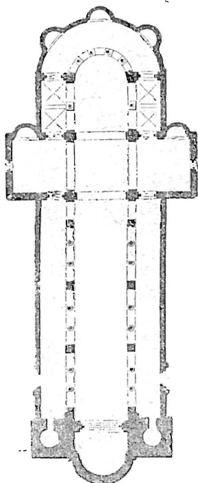
Рис. 17-й. Планъ храма романо-византїскаго (въ Гильдесгеймѣ).
