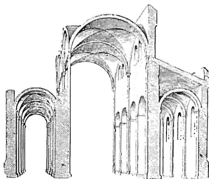
Рис. 18-й. Своды романо-византїскіе.
