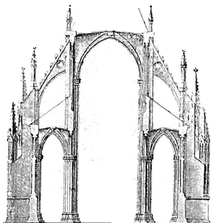
Рис. 21-й. Поперечный разръзъ го- тического храма.
